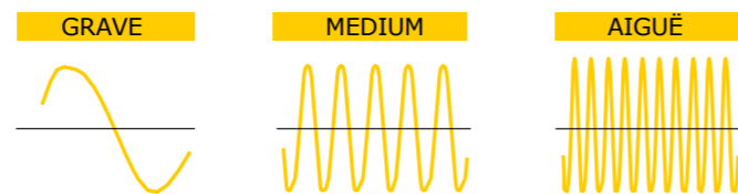
La fréquence exprime le nombre de vibrations par seconde.
